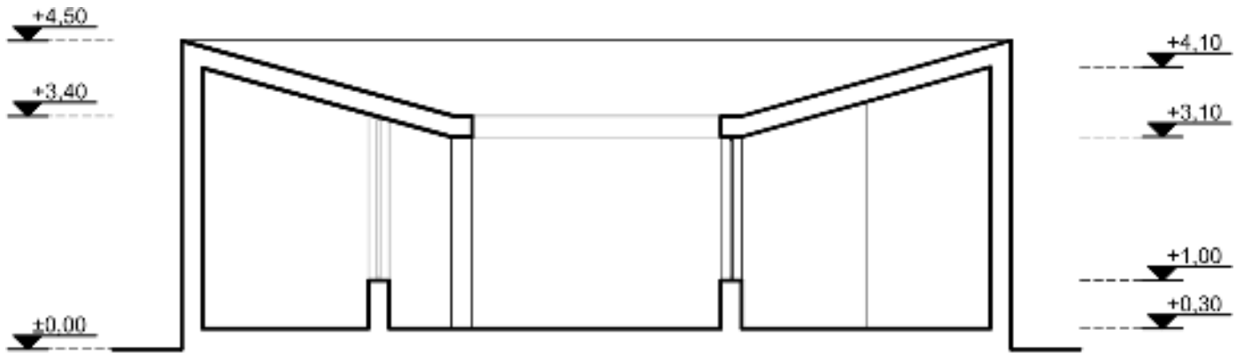
ΤΟΜΗ Α-Α
